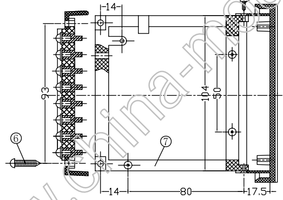
线路板支架安装示意图
