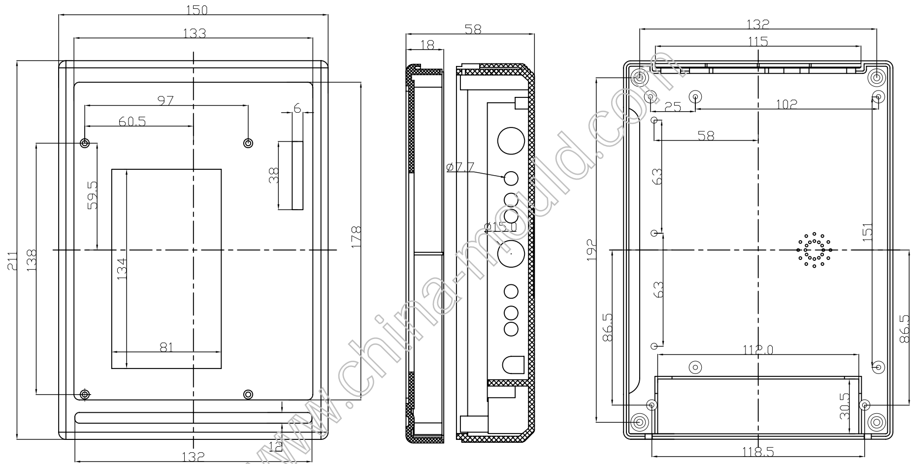
下盖正视图
