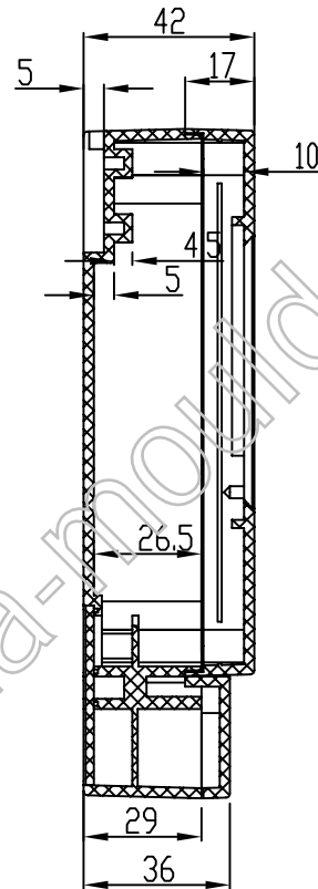
A-A
