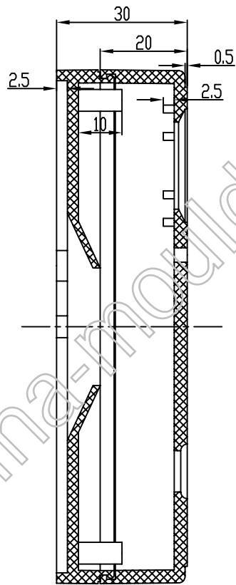
A-A
