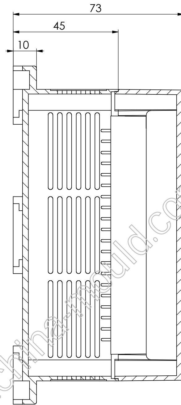
剖面 A-A
