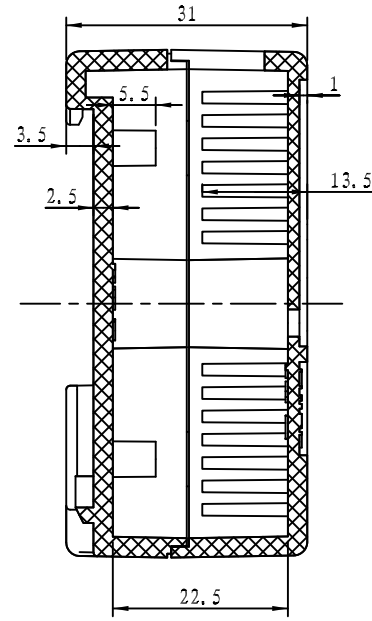
剖面 B-B
