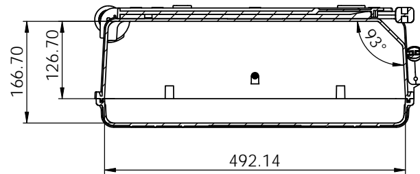
剖面 C-C
