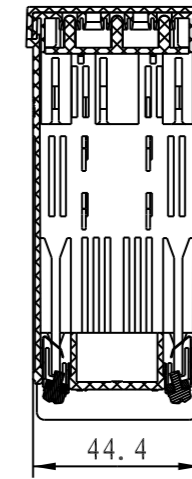
剖面 A-A
