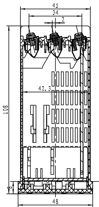
截面 A-A
